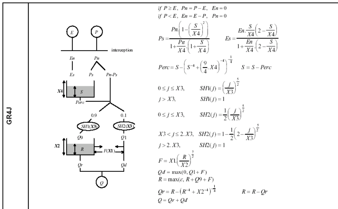
FIGURE 3.2 – Architecture du modèle global : GR4J (Mouelhi, 2003, Mouelhi et al. 2006)
