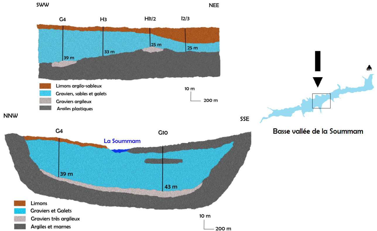
FIGURE 5.2 – Coupe géologique au Sud d’El Kseur (Kessasra, 2014)
