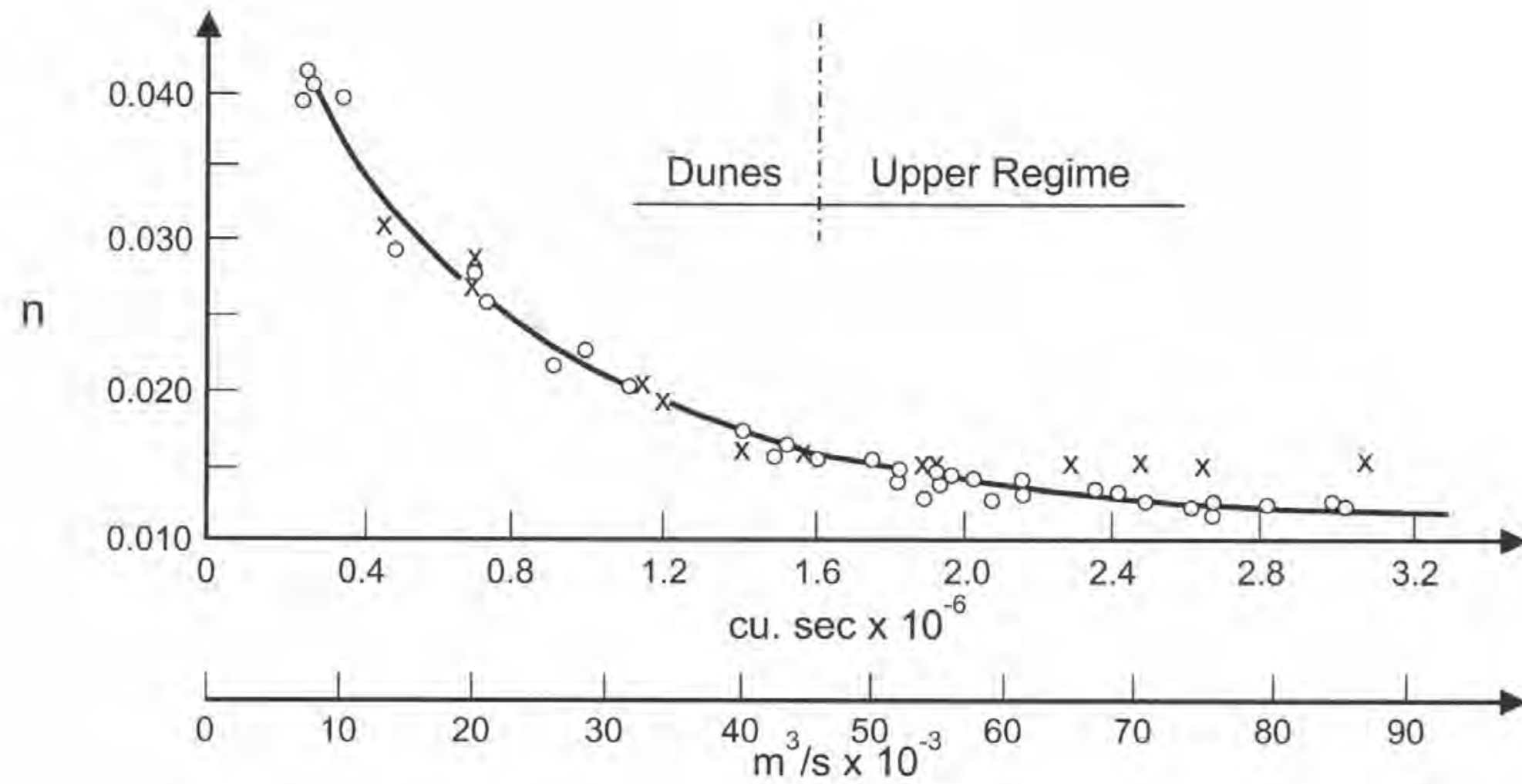
Variation de n = 1/K au cours d'une crue.
